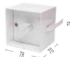
Luftklappengriff quadratisch, vertieft – Design 1
