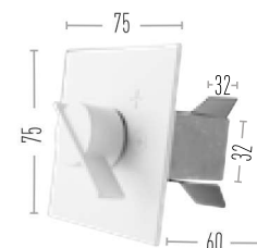
Luftklappengriff quadratisch, einf. Ausführung – Design 1
